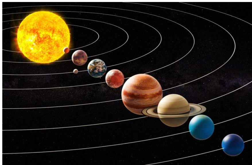
Мегамир. Солнечная система
