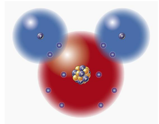
Микромир. Атом водорода и молекула воды
